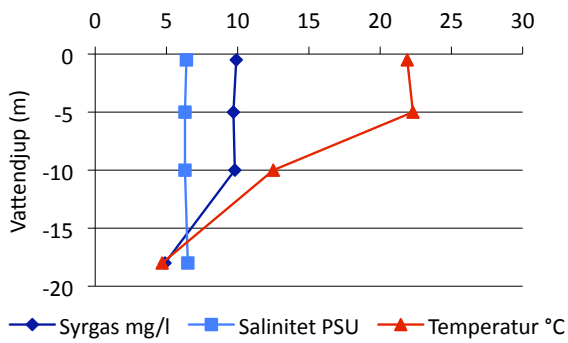
Va03 Valdemarsviken inre 6/7 2009
