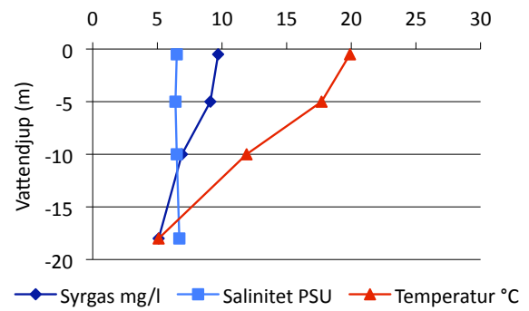
Va03 Valdemarsviken inre 13/8 2009
