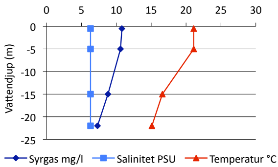
Va05 Valdemarsviken yttre 6/7 2009
