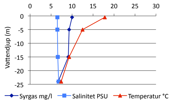
Va05 Valdemarsviken yttre 13/8 2009
